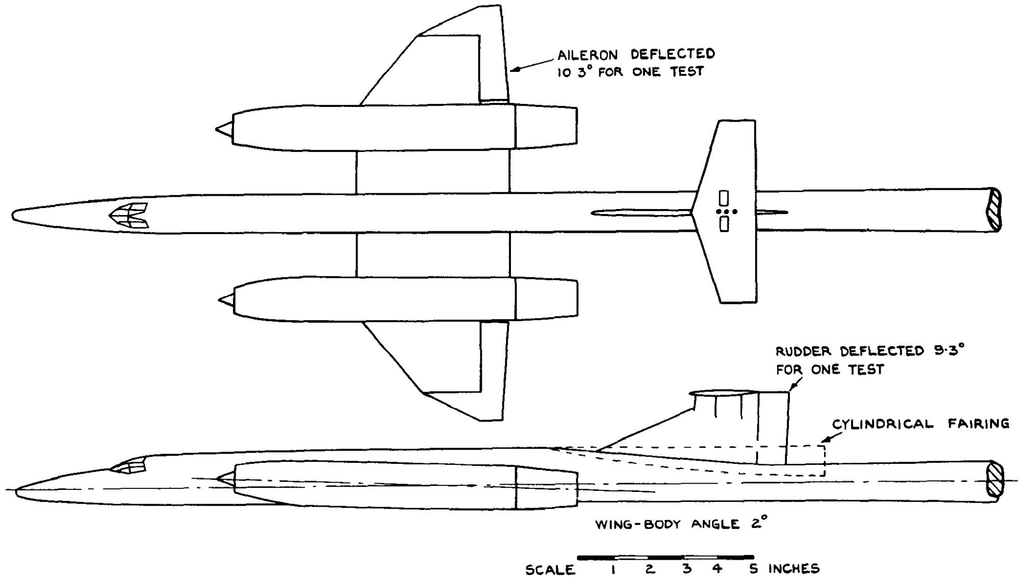
FIG. I. G.A. OF MODEL A.
