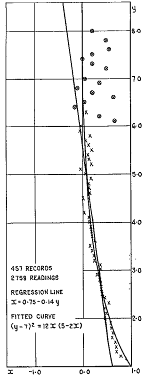
FIG. 4. Swift Mk. 1.
