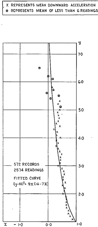
FIG. 7. Meteor NF11.
