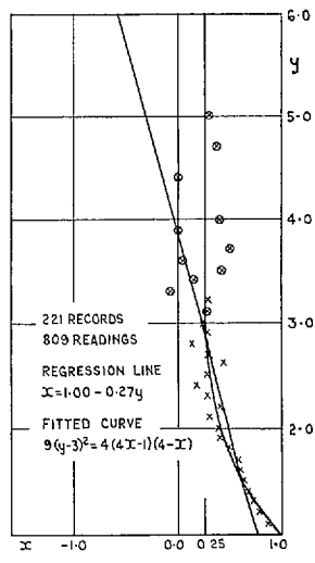
FIG. 13. Gannet A/S Mk. 1 .
