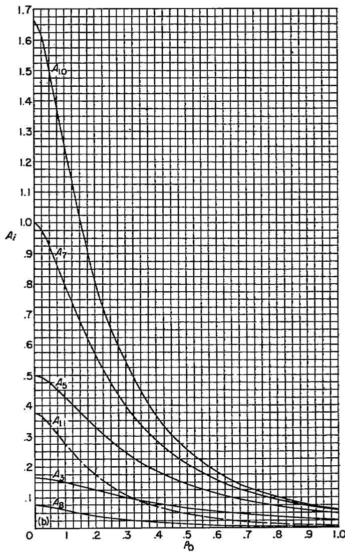
(b) A_i
