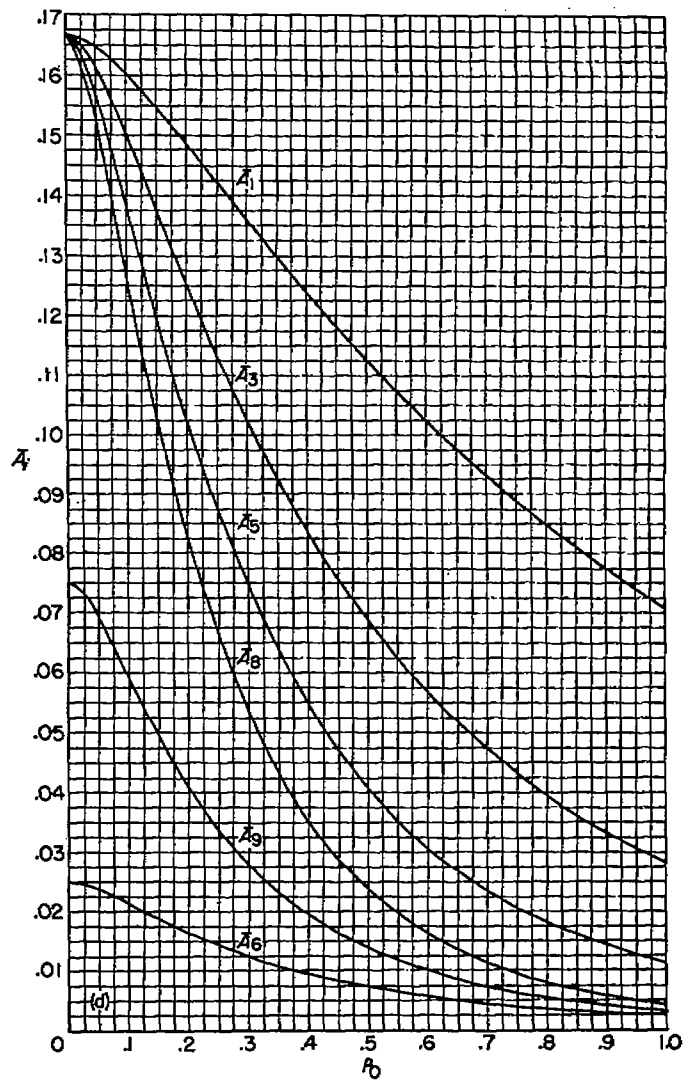
(d) \bar{A}_i .
