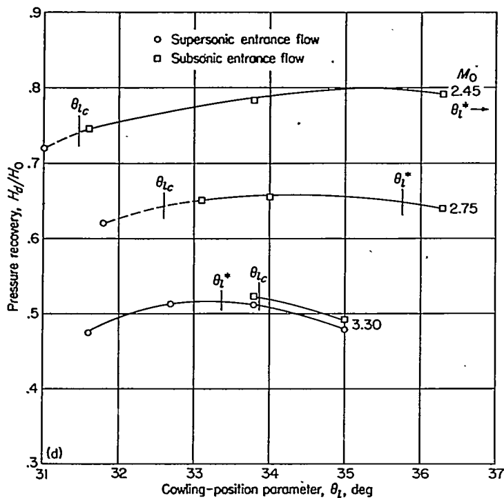
(d) 4^\circ, 7^\circ cowling; D_b/D_t=0.834 ; \theta_c=25^\circ . FIGURE 18.—Continued.
