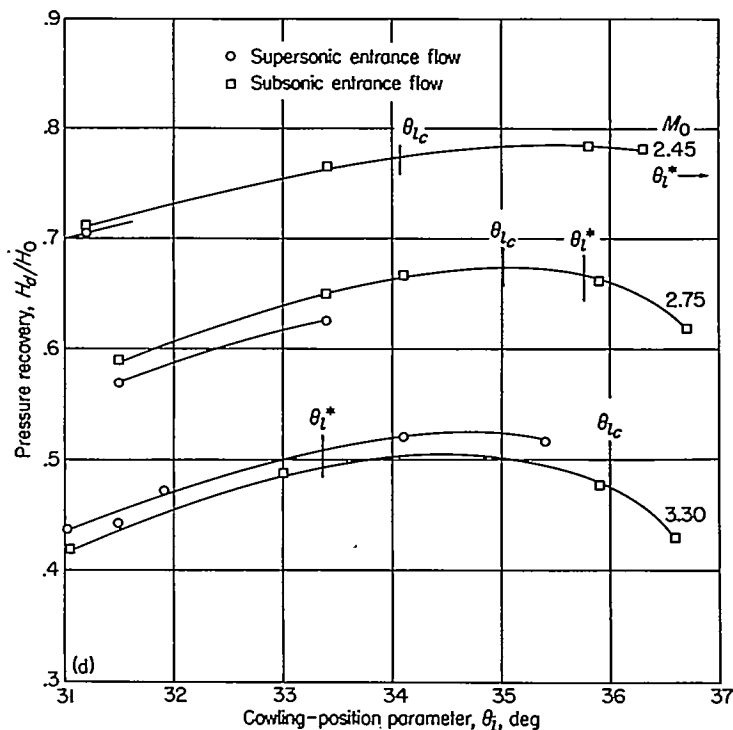
(d) 7^\circ, 10^\circ cowling; D_b/D_i=0.817 ; \theta_c=25^\circ . FIGURE 19.—Continued.
