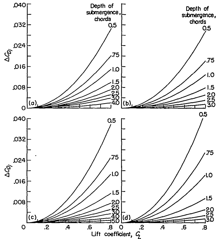
(a) A=10 ; tank no. 1. (b) A=10 ; tank no. 2. (c) A=6 ; tank no. 1. (d) A=4 ; tank no. 2.
