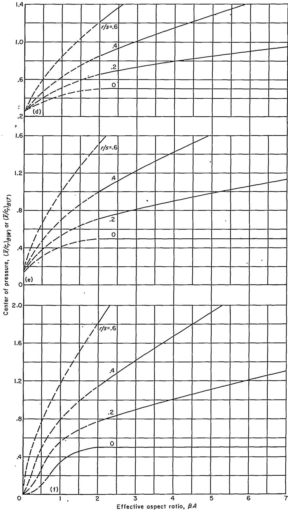
(d) No midchord sweep, \lambda=0 . (e) No midchord sweep, \lambda=1/2 . (f) No midchord sweep, \lambda=1 .
