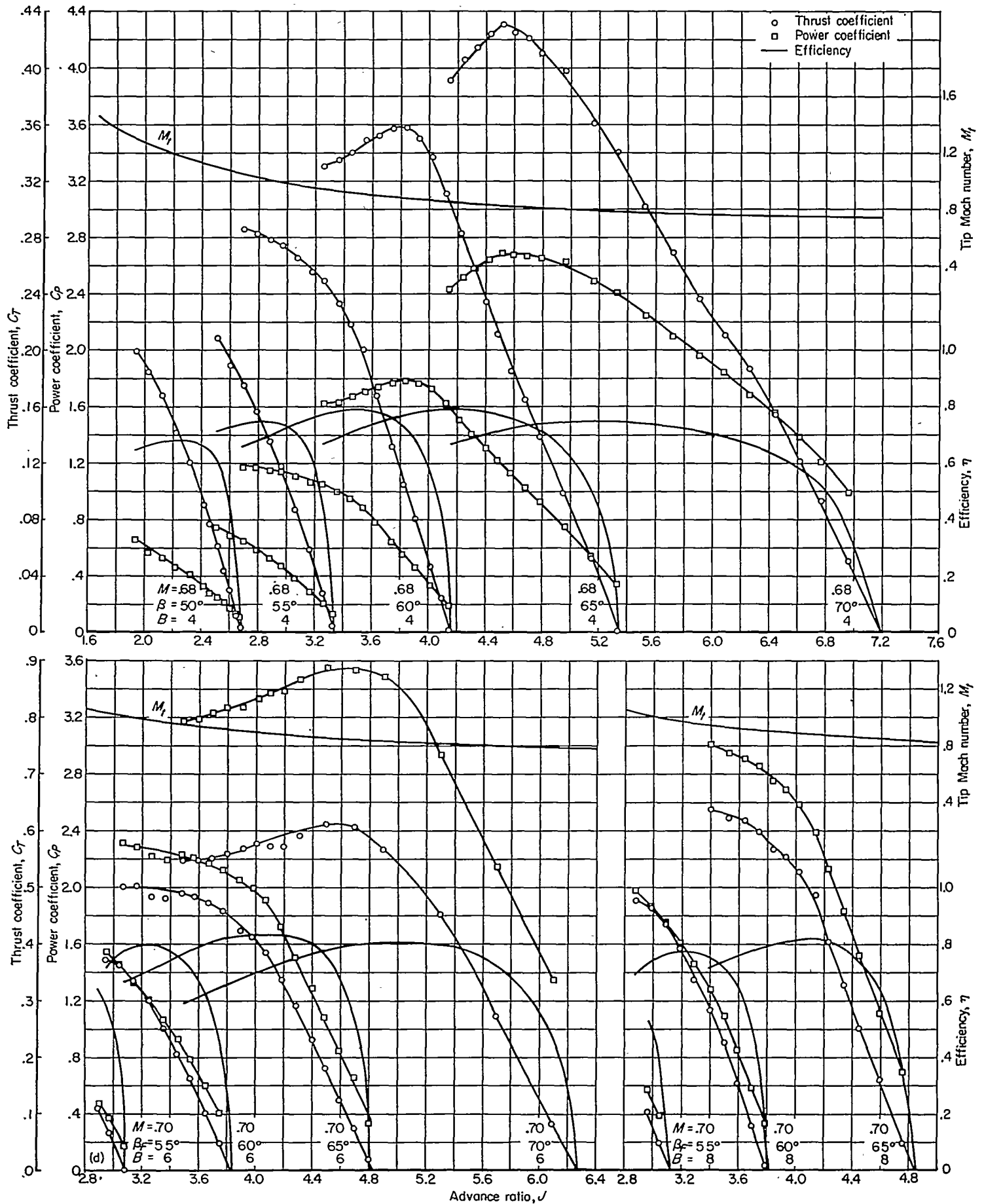
(d) M_t \approx 0.70 FIGURE 7.—Continued.
