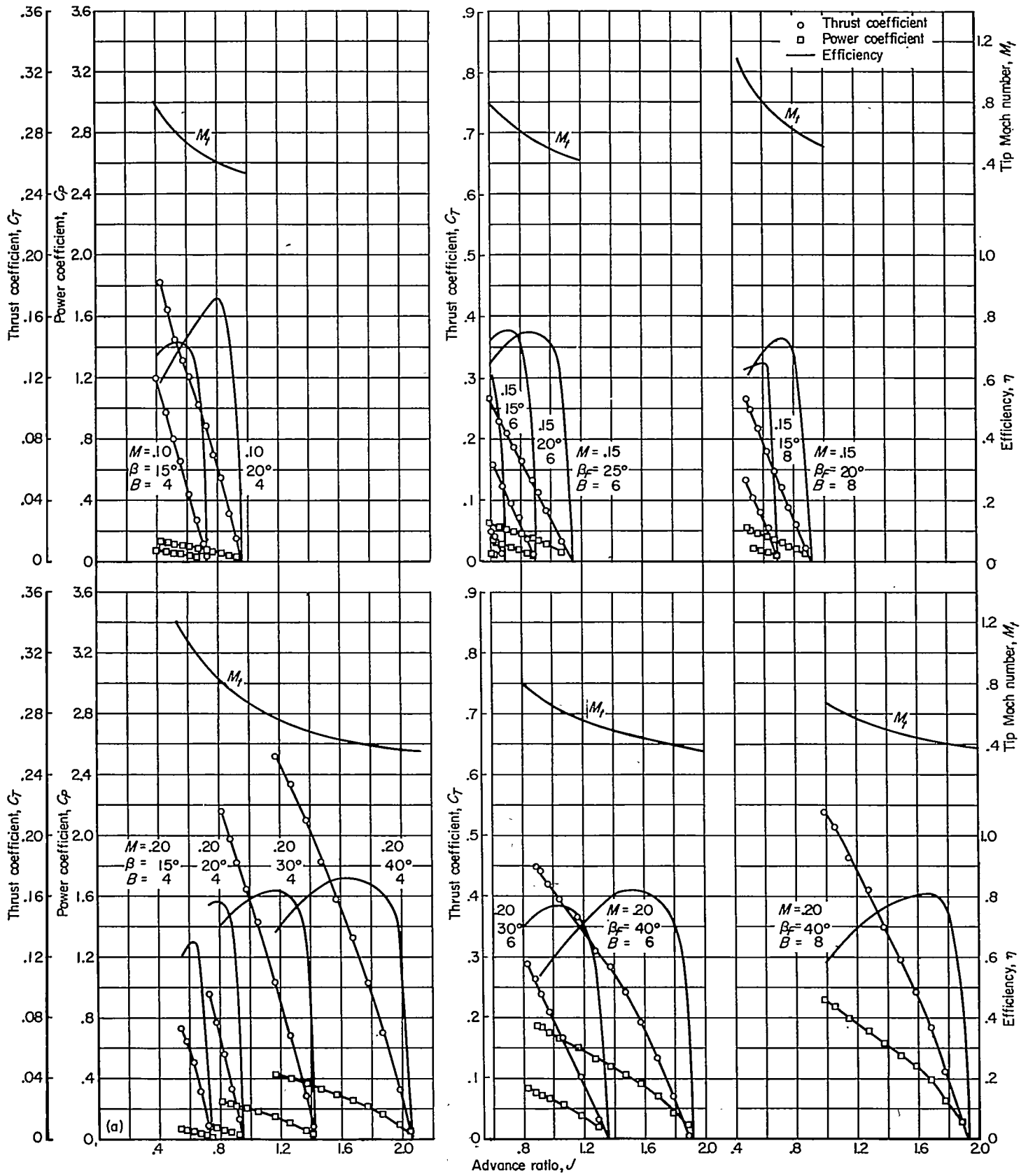
(a) M \approx 0.10 to 0.20
