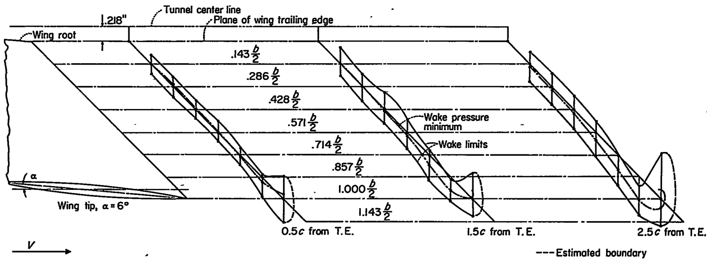
(c) Scale: Inches
