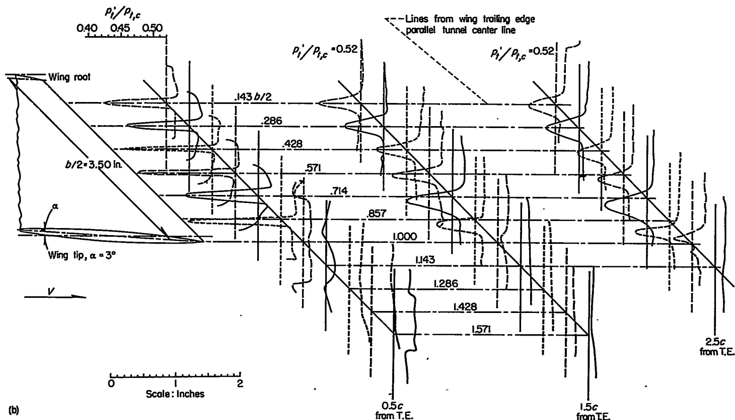
(b) \alpha = 3^\circ .
