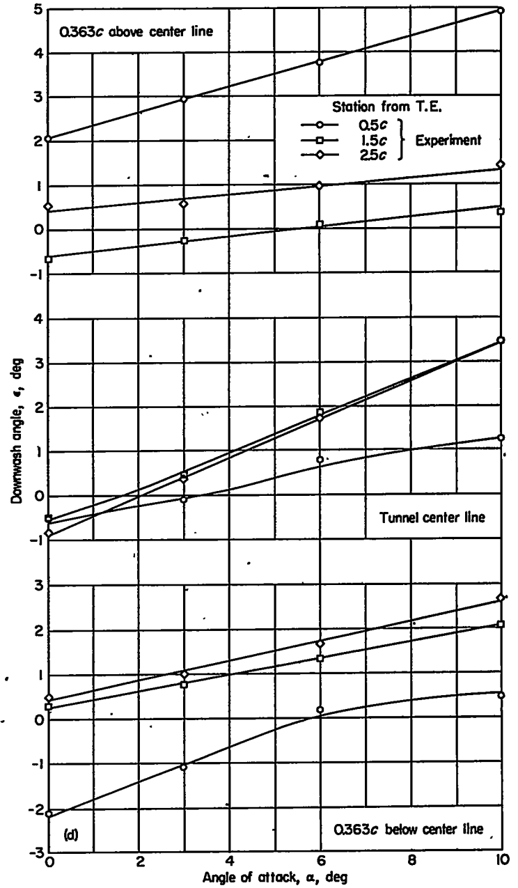
(d) Spanwise station, 0.714\frac{b}{2} .
