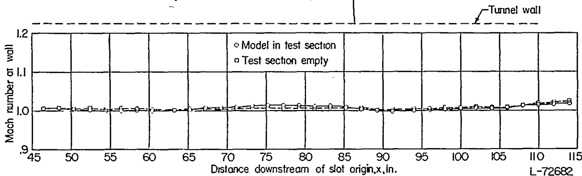
(d) M_0 = 1.008 .
