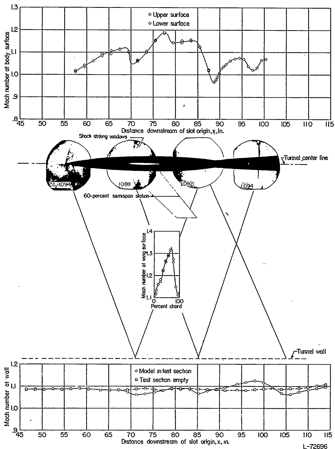
(d) M_o=1.088 .
