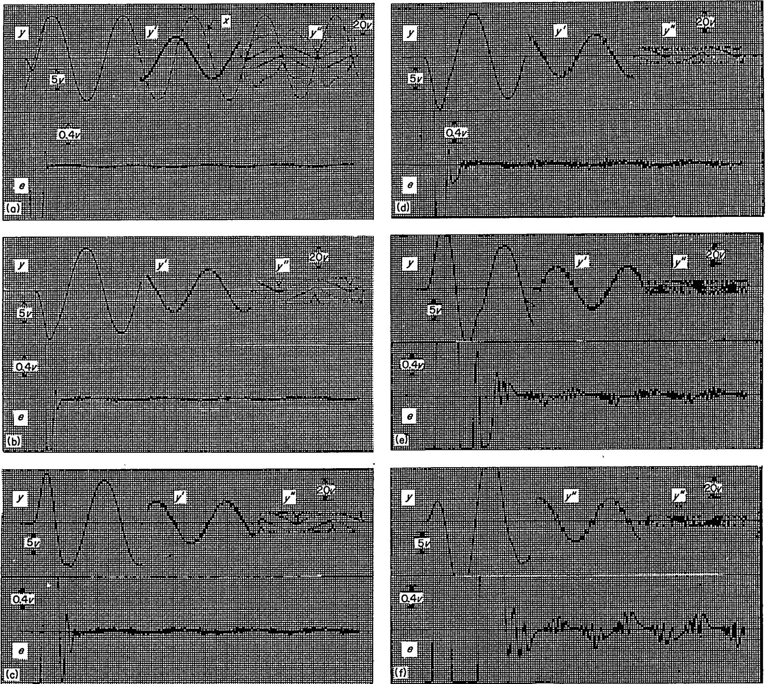
(a) Nonlinear system; no y'' limit. (b) Nonlinear system; \pm 12 -volt y'' limit. (c) Nonlinear system; \pm 9 -volt y'' limit. (d) Nonlinear system; \pm 7\frac{1}{2} -volt y'' limit. (e) Nonlinear system; \pm 6 -volt y'' limit. (f) Nonlinear system; \pm 4\frac{1}{2} -volt y'' limit.
