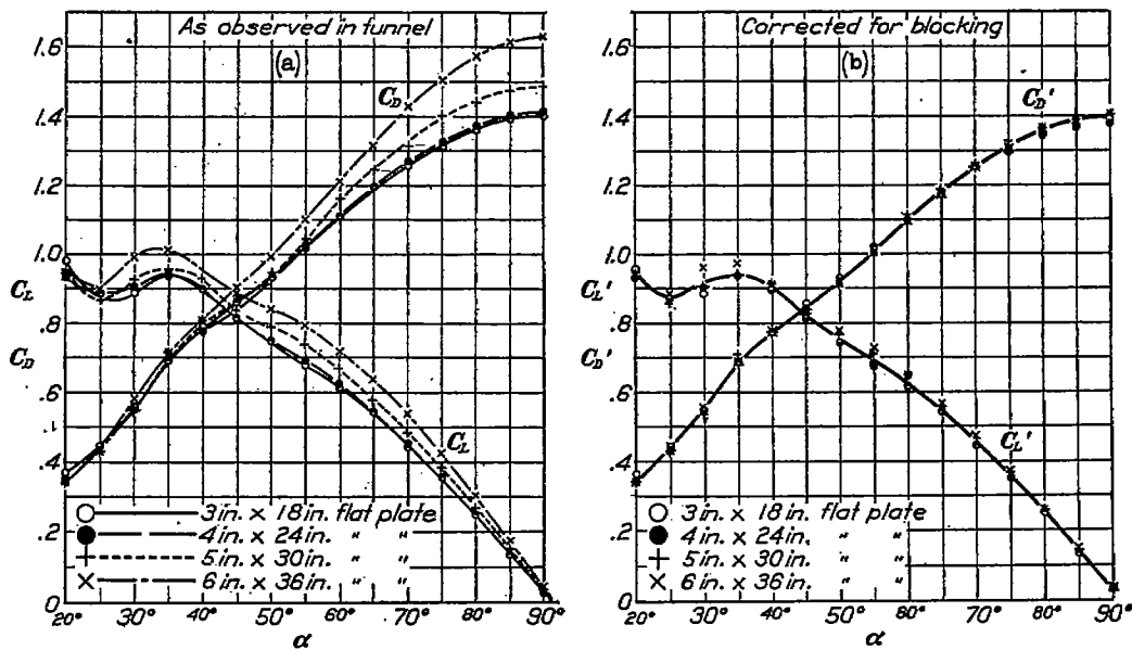
FIGURE 57.—Flat plates. A. R. 6
