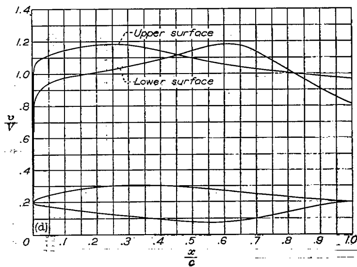
(d) NACA 836A110 airfoil.
