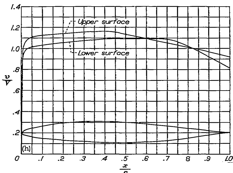
(h) NACA 847B110 airfoil.
