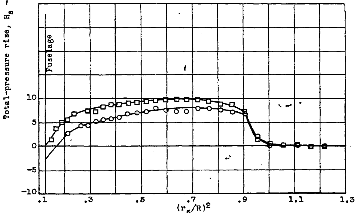
(b) C_p , 0.30; J , 2.36; M_0 , 0.40; M_t , 0.67.
