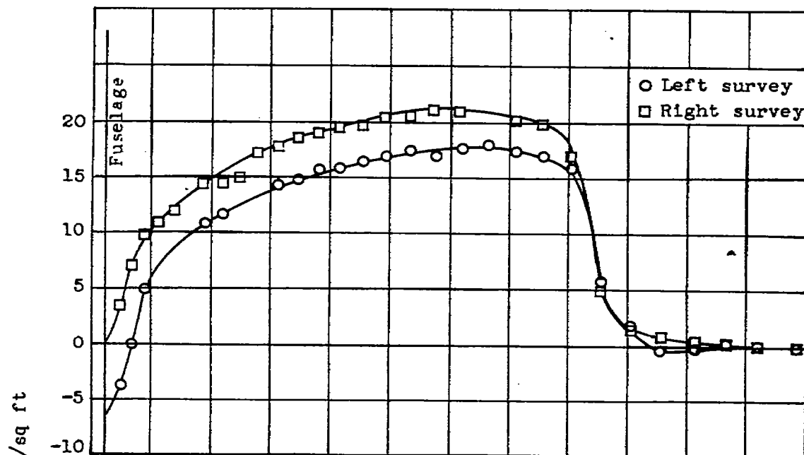
(d) C_p, 0.61 ; J, 2.36 ; M_o, 0.51 ; M_t, 0.85 .
