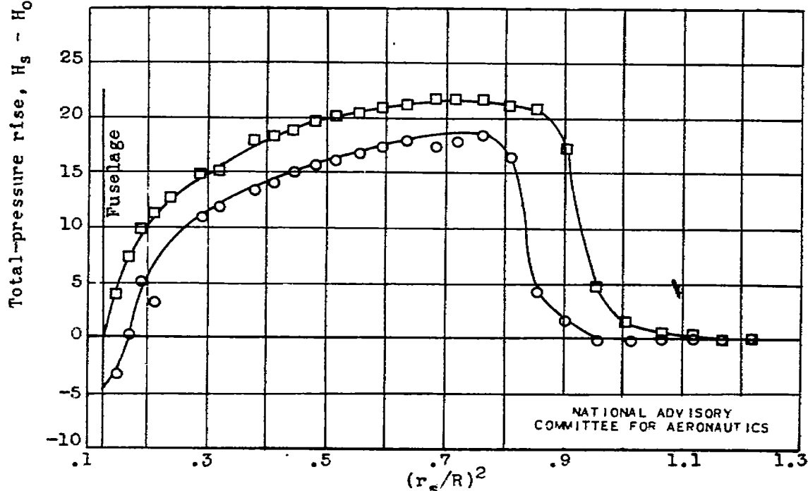
(e) C_p, 0.60 ; J, 2.25 ; M_o, 0.48 ; M_t, 0.83 .
