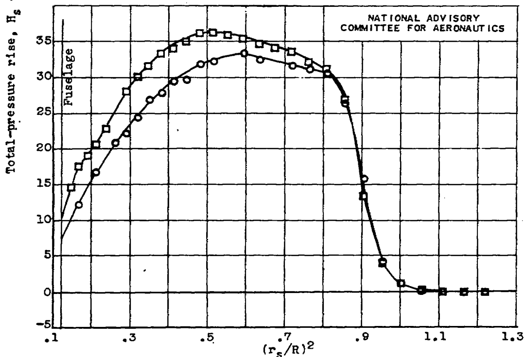
(d) C_p , 0.40; J , 1.01; M_0 , 0.29; M_t , 0.94.
