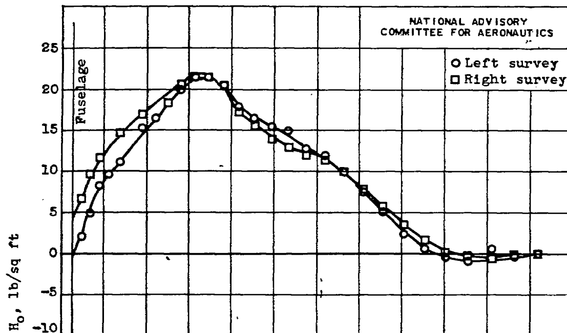
(d) C_p , 0.71; J , 1.66; M_o , 0.37; M_t , 0.80.
