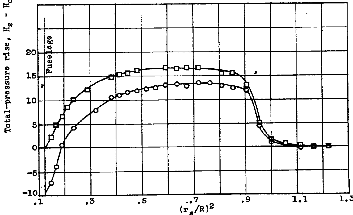
(d) C_p, 1.01 ; J, 3.04 ; M_o, 0.51 ; M_t, 0.73 .
