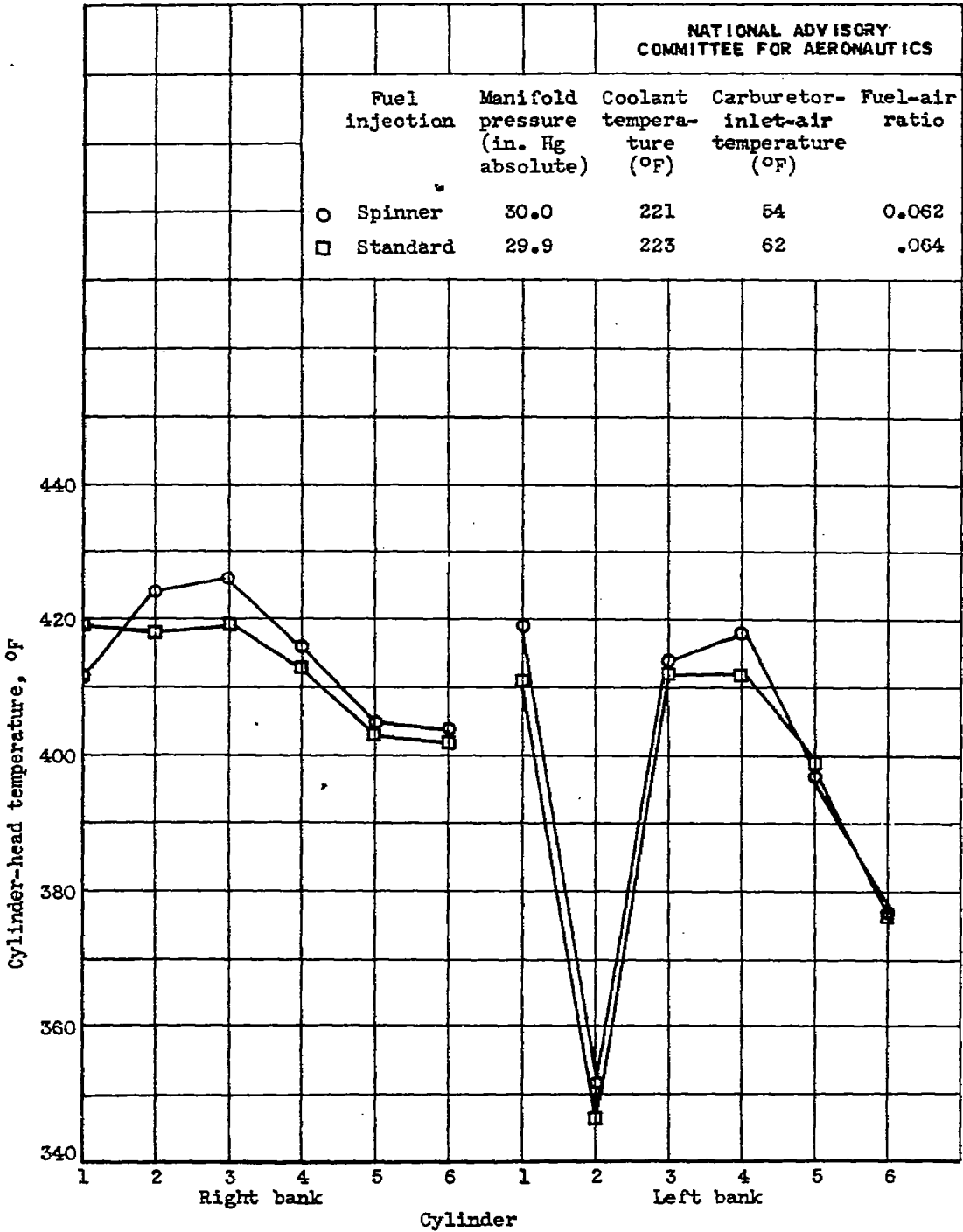
(d) Manifold pressure, 30 inches of mercury absolute.
