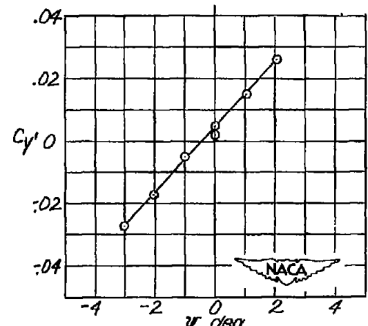
(d) \alpha = -2.85^\circ , \psi , deg
