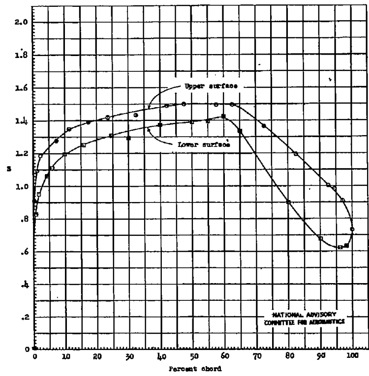
(d) \alpha_0 = 0^\circ .
