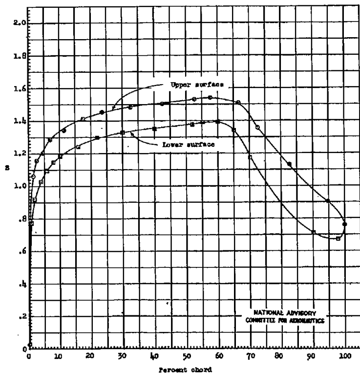
(d) \alpha_0 = 0^\circ Figure 7.- Continued.
