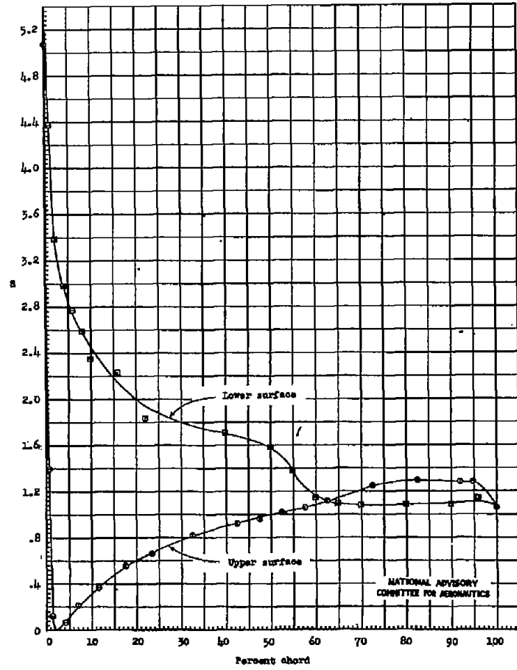
(d) \alpha_0 = -12.2^\circ Figure 4.- Continued.
