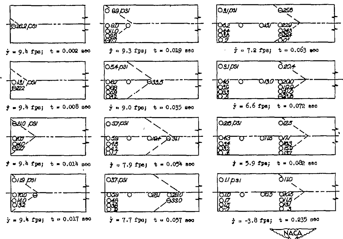
(b) Run 7: \tau = 15^\circ ; x_0 = 90.9 feet per second; \dot{y}_0 = 9.4 feet per second.
