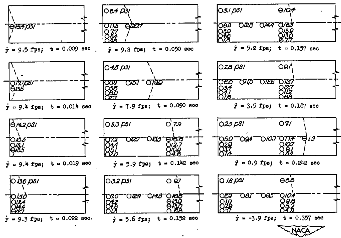
(d) Run 21: \tau = 45^\circ ; \dot{x}_0 = 50.5 feet per second; \dot{y}_0 = 9.5 feet per second.
