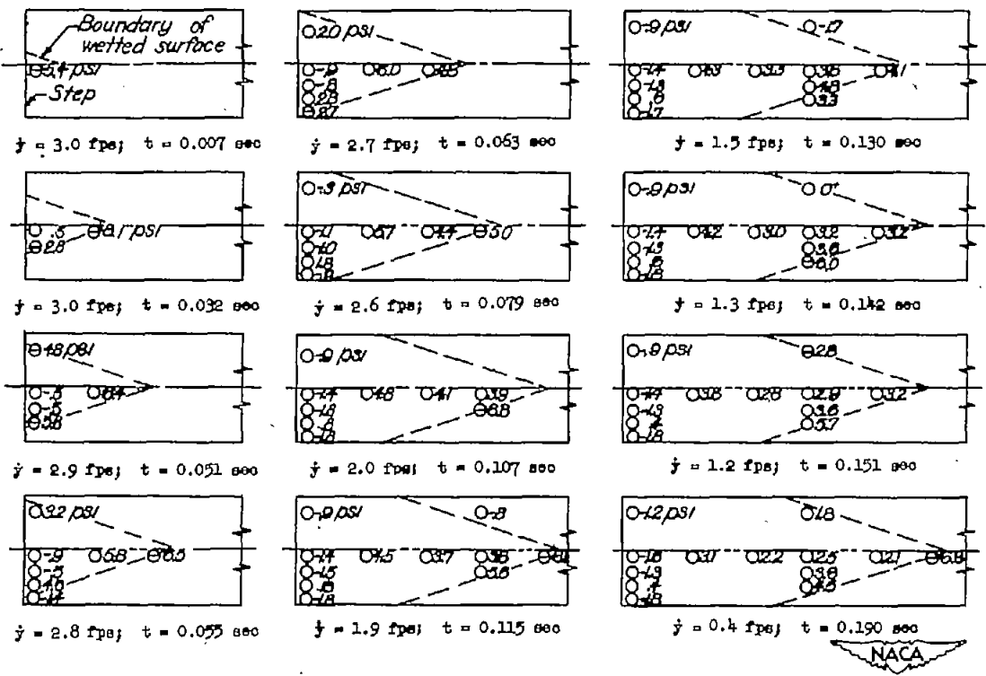
(a) Run 2: \tau = 6^\circ ; \dot{x}_0 = 89.3 feet per second; \dot{y}_0 = 3.0 feet per second.
