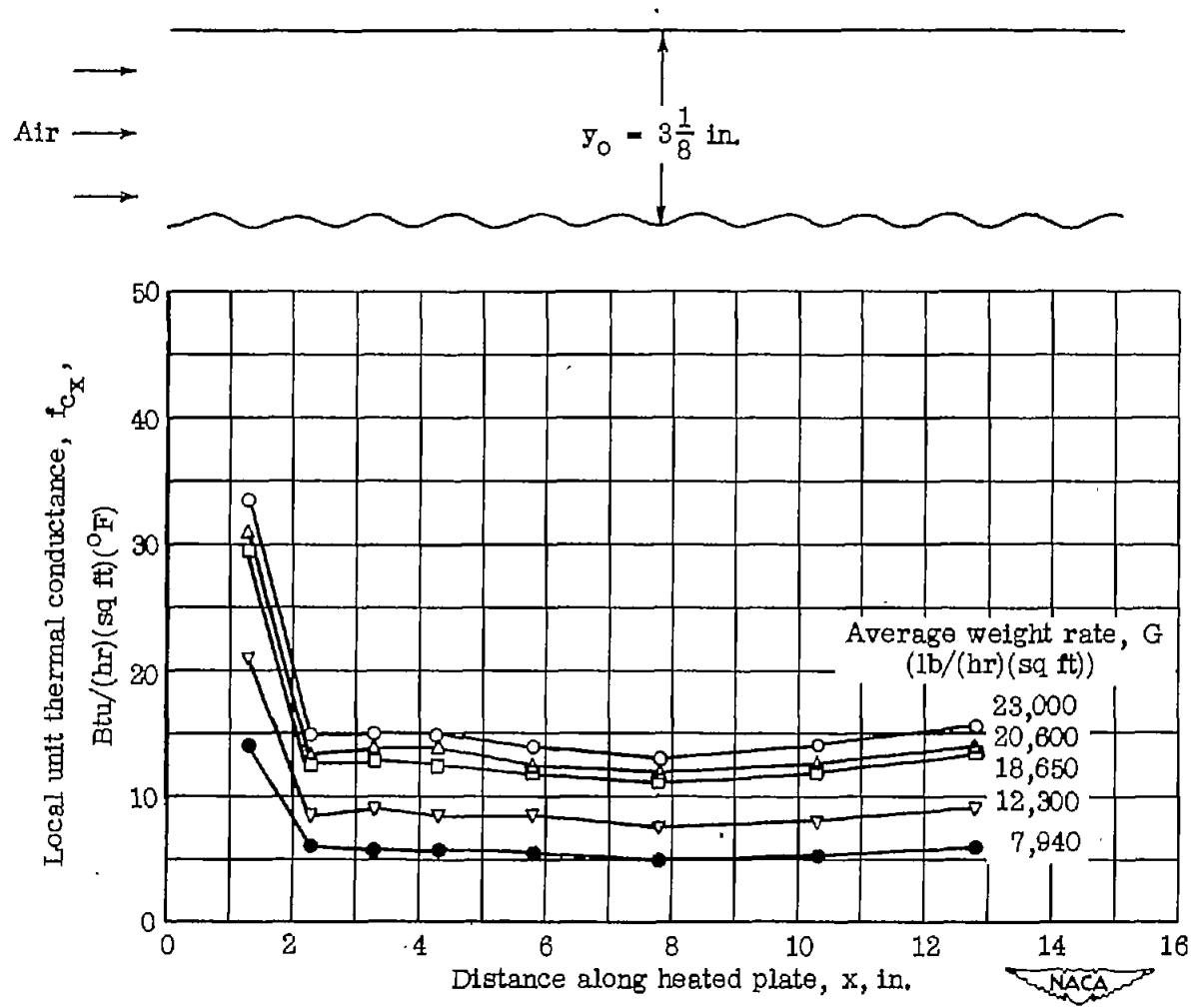
(d) Small wave plate at y_0 = 3\frac{1}{8} inches.
