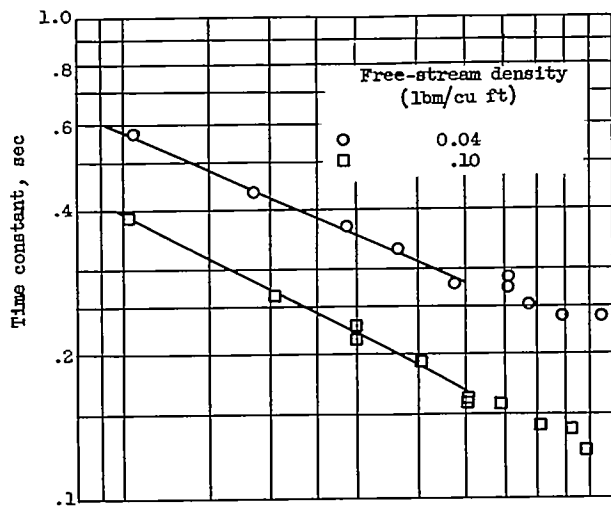
(d) Probe D; iron-constantan; diameter, 0.0160 inch.
