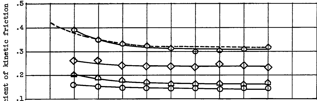
(e) Tetralin.
