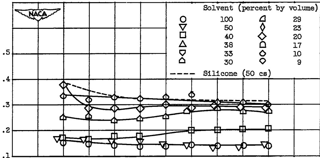
(d) Cyclohexene.
