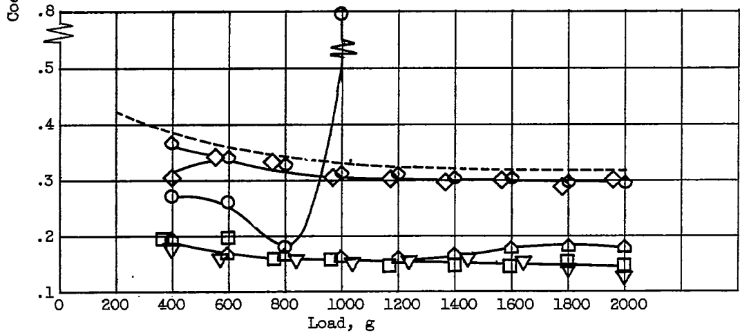
(f) Toluene.
