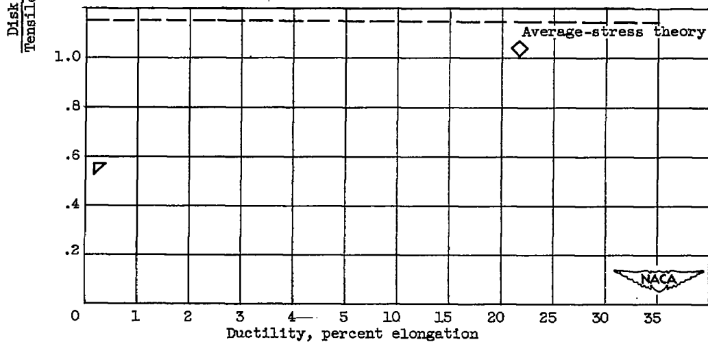
(d) Disks with four 3/8-inch-diameter eccentric holes.
