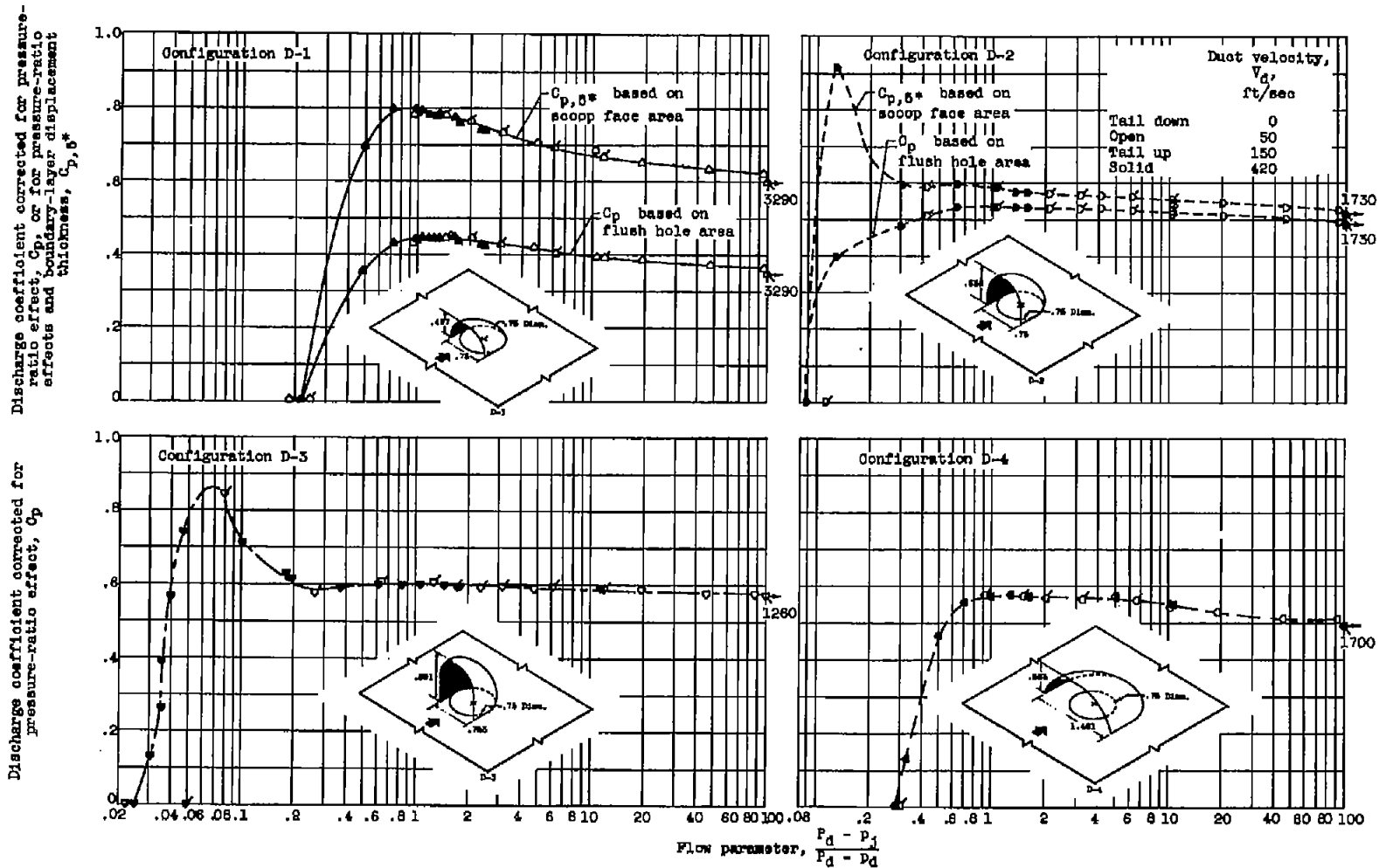
(d) Scoops over circular holes.
