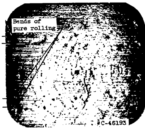
(d) Ball surface; X75; 210 \times 10^6 stress cycles.
