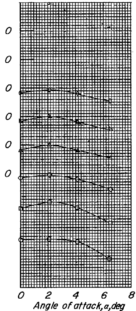
(d) 60-4-.6-006 wing.
