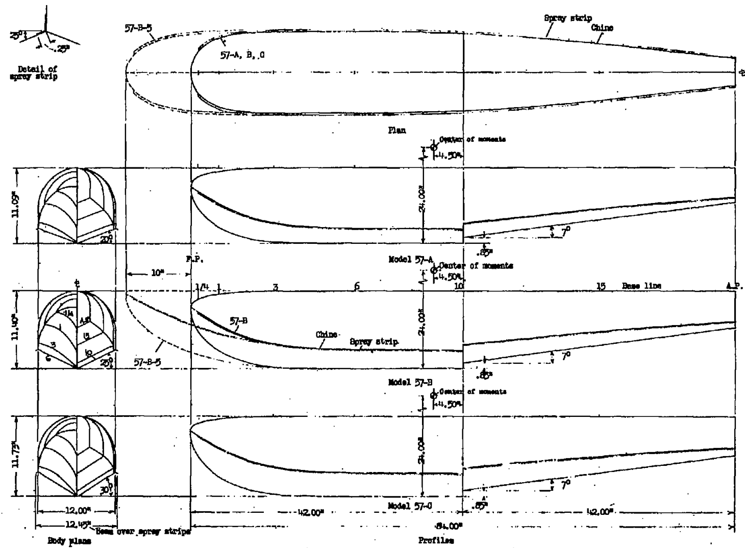
Fig. 1 - Lines of N. A. C. A. model 57 series.
