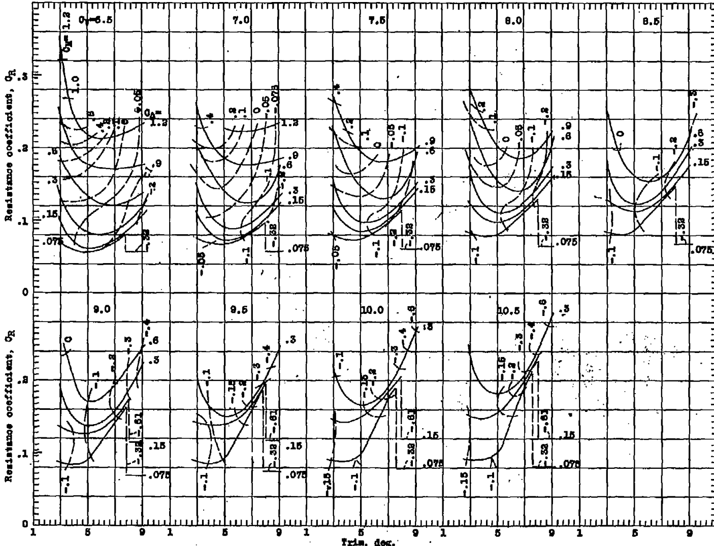
Figure 14d.- Model 57-B.
