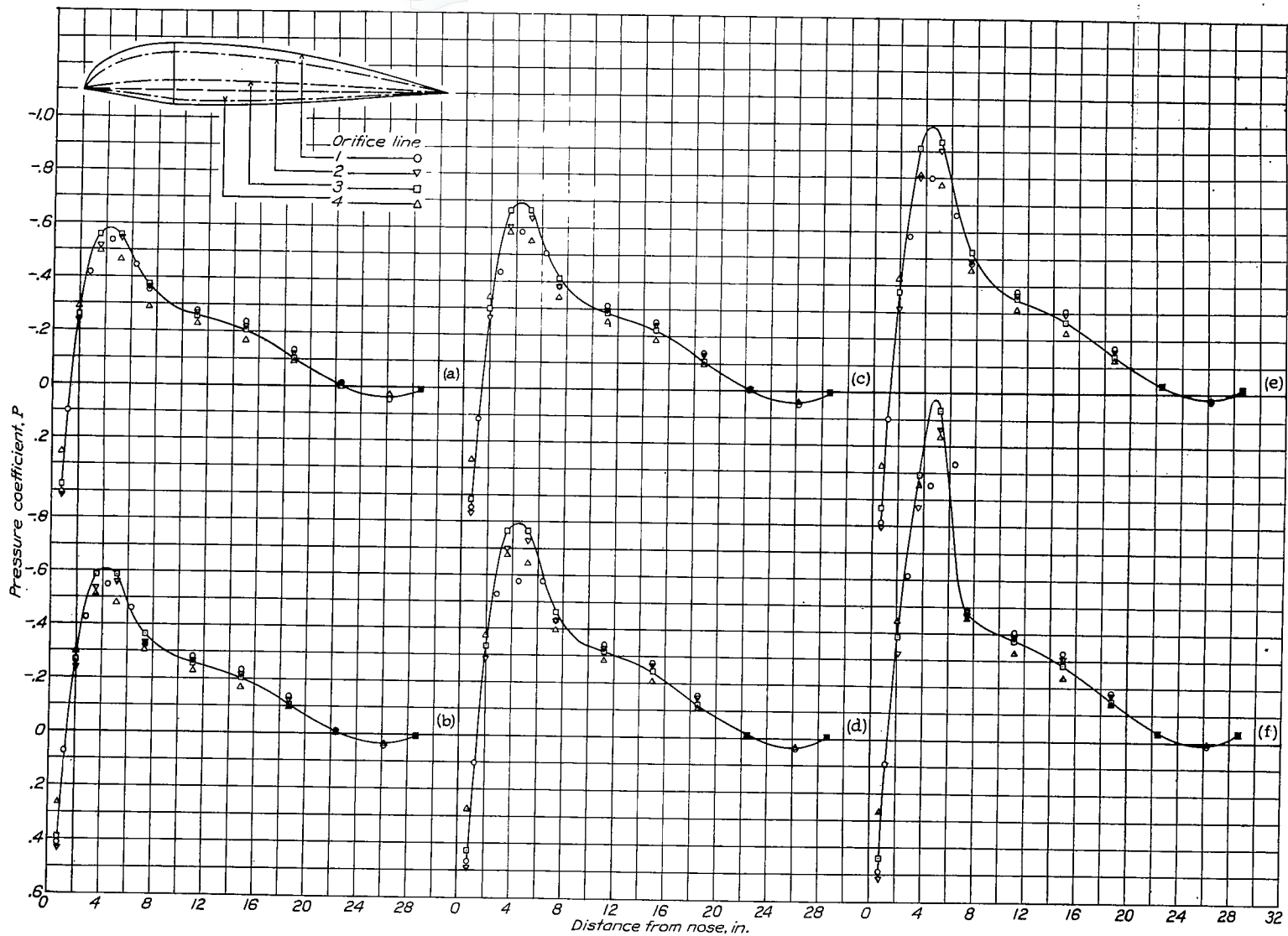
(a) M, 0.199 (b) M, 0.340 (c) M, 0.535 (d) M, 0.632 (e) M, 0.689 (f) M, 0.716
