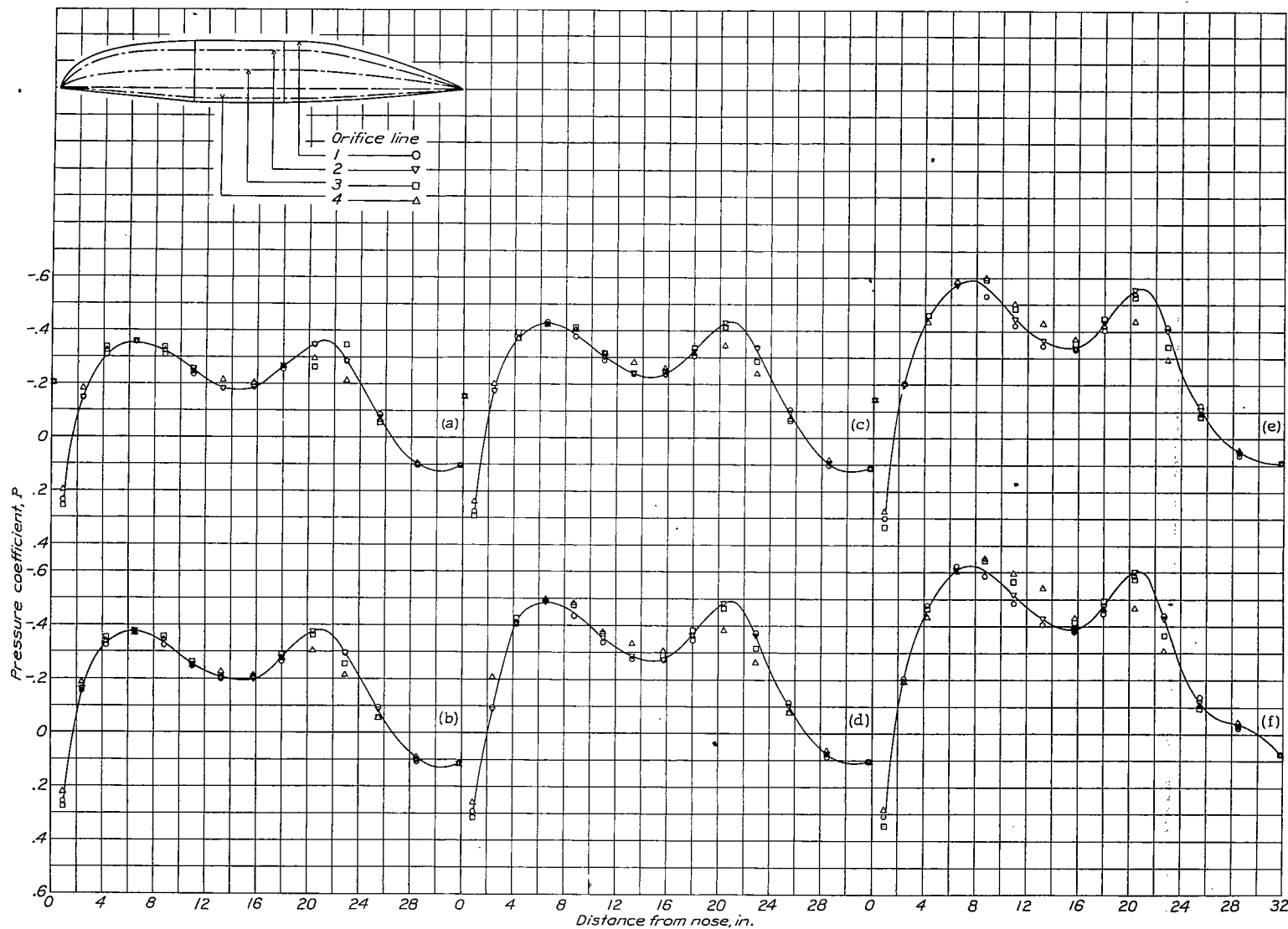
(a) M , 0.195 (b) M , 0.342 (c) M , 0.539 (d) M , 0.630 (e) M , 0.692 (f) M , 0.712
