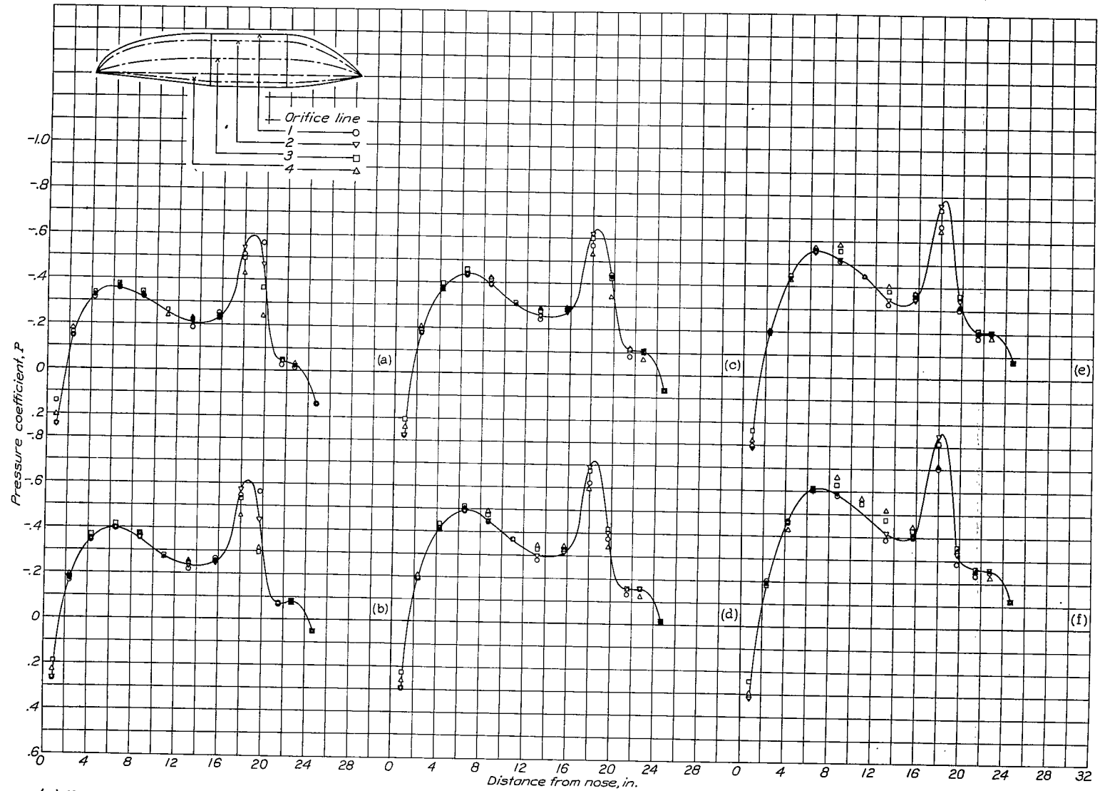
(a) M , 0.197 (b) M , 0.433 (c) M , 0.537 (d) M , 0.627 (e) M , 0.681 (f) M , 0.707
