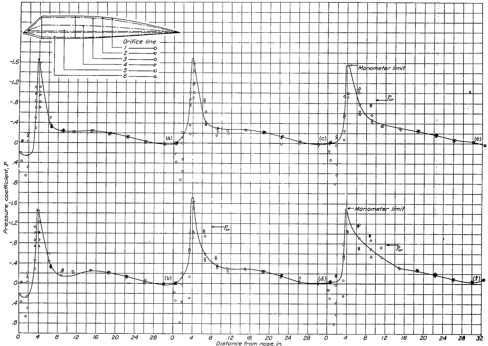
(a) M, 0.192 (b) M, 0.341 (c) M, 0.535 (d) M, 0.631 (e) M, 0.682 (f) M, 0.962
