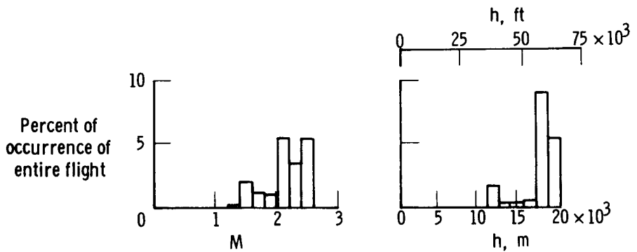
(d) Cruise.
